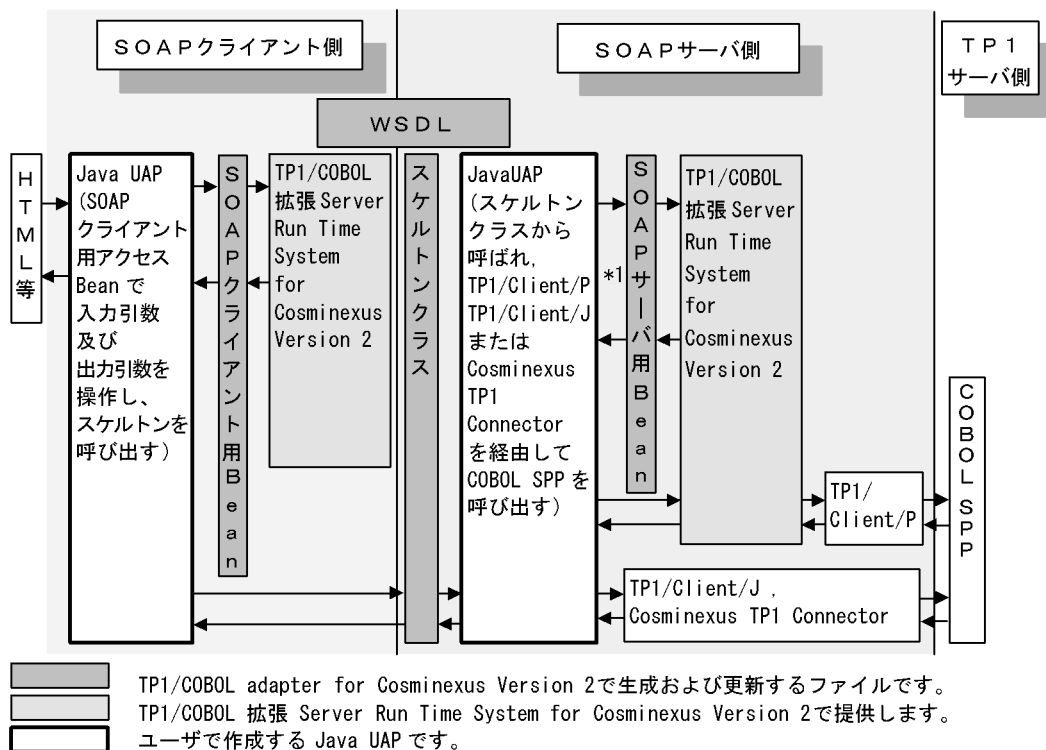
図 10-1 SOAP サービス使用時の処理の流れ
